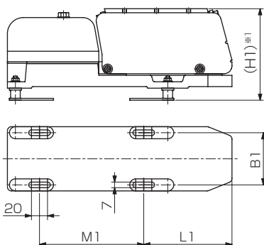
寸法表 Dimension table 単位: mm Unit: mm
