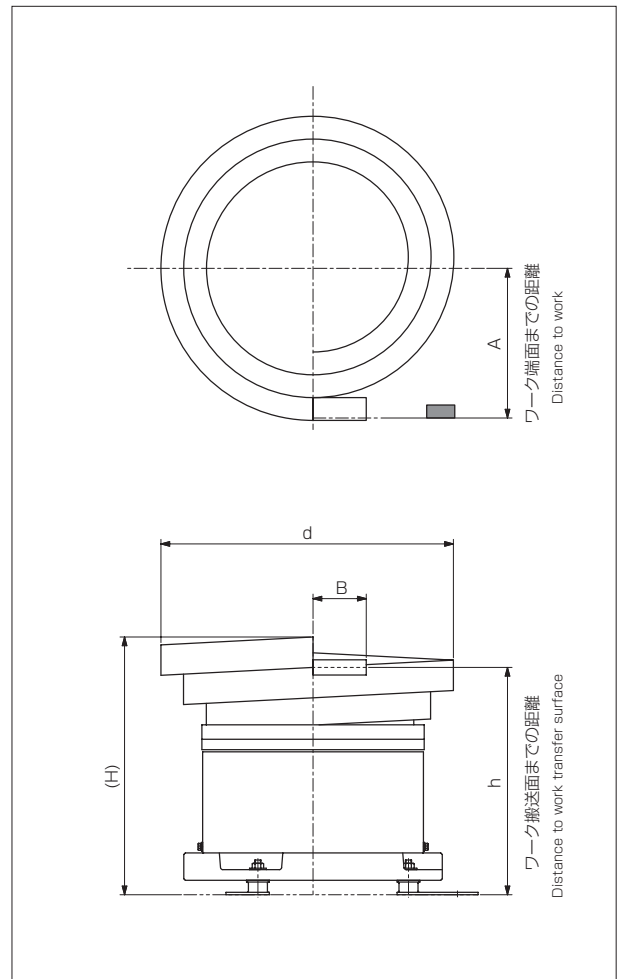
段付寸法表 Dimension table of cascade type 単位: mm Unit: mm
